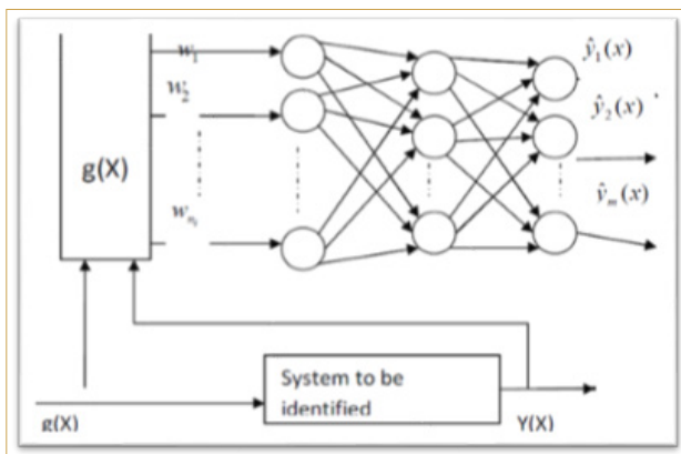
شكل (٤) الهيكل العام للشبكة العصبية متعددة الطبقات ذات التغذية الراجعة
