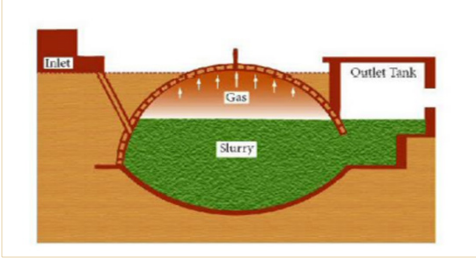
الشكل ذو العدد (٧) : مخمر دينباند هو
